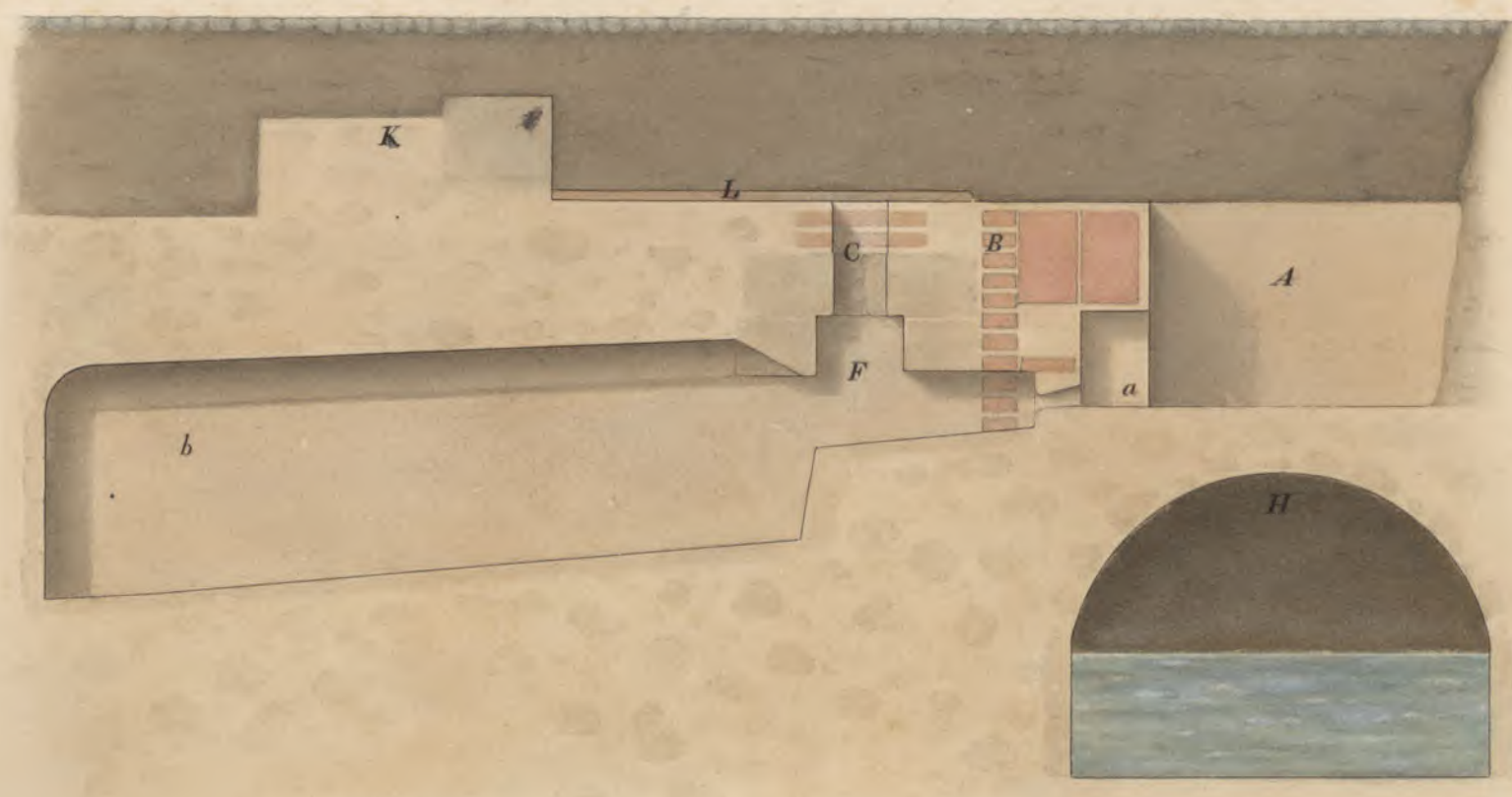
Córtice tirado sobre o centro do cano das thermas na linha P,Q.
